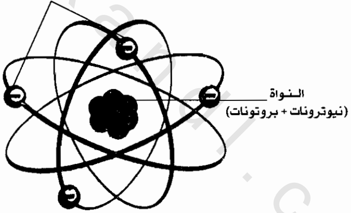
رسم تخطيطي لذرة عنصر
