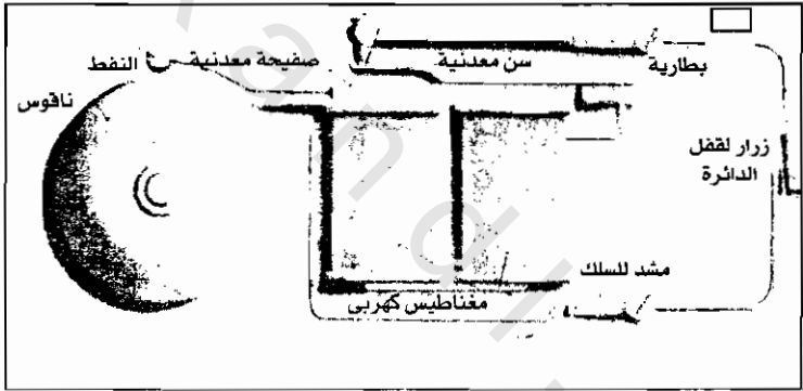
المسار الذي يتخذه التيار الكهربى عند فقل الدائرة
