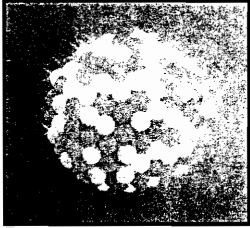
الإلكترونات سالبة الشحنة
