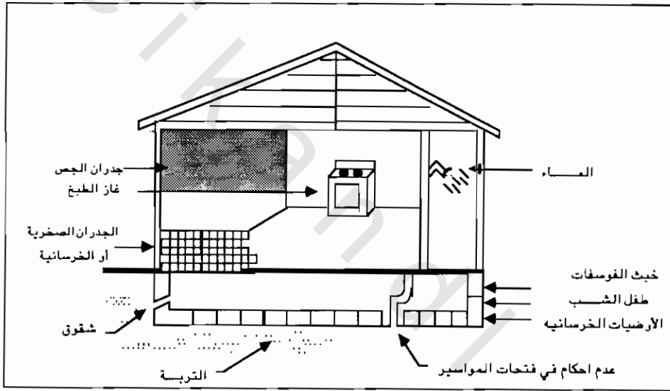
شكل (٤ - ٢) مصادر الرادون في المساكن (٨) . .
