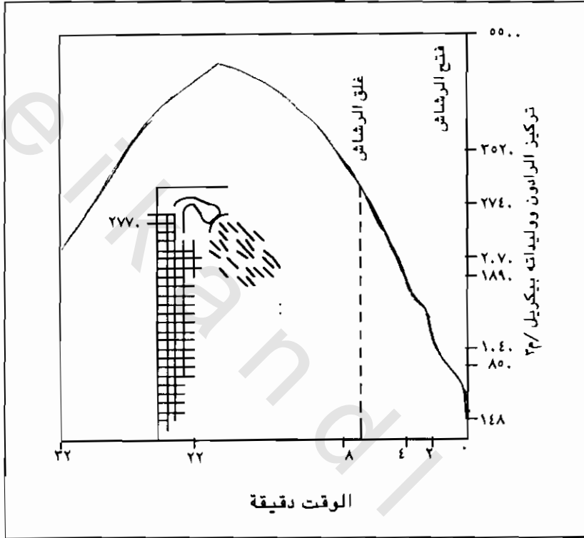
شكل (٤ - ٥) تركيز الرادون ووليداته في الهواء الداخلي لحمام خلال الاستحمام برشاش دافئ لمدة سبع دقائق في مسكن بكندا . وكان تركيز الرادون بالماء ٤٤٠٠ بيكريل / م ٣ (١٠).
