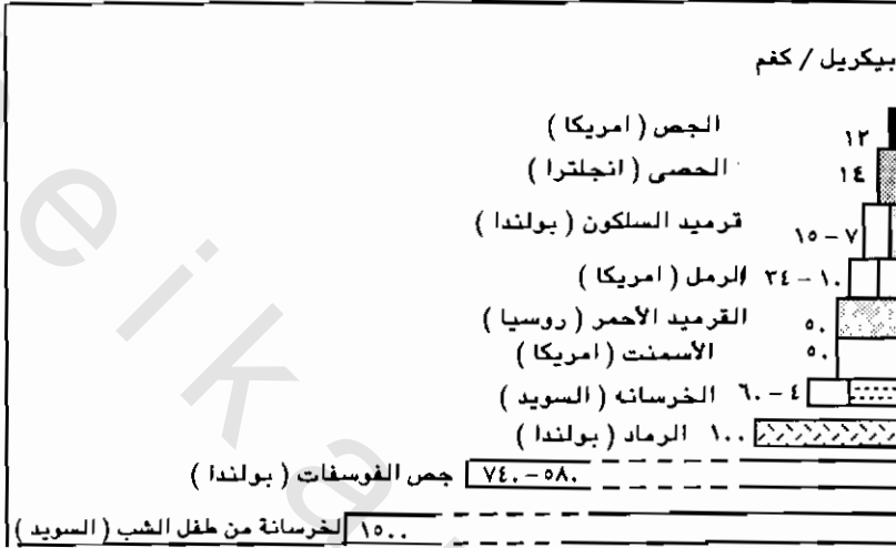
شكل (٤ - ٣) النشاط الإشعاعي المعتاد للراديوم في بعض مواد البناء (٤).
