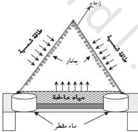
شكل (9): مبدأ عمل وحدة تحليه شمسية
