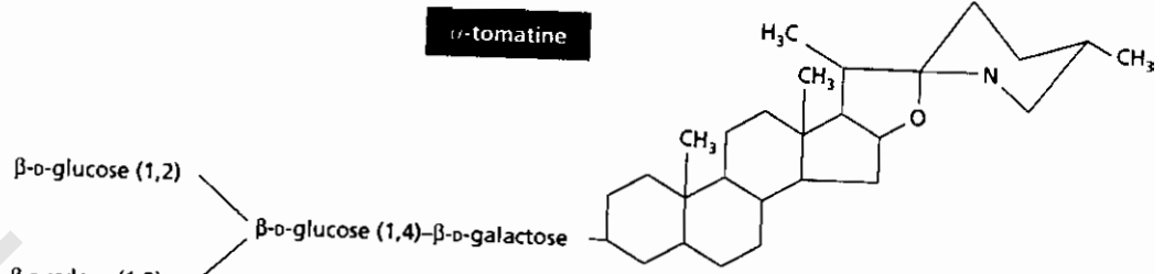
شكل (٥٧٤) : تركيب الفانوماتين.
