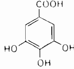
Gallic acid شكل (٢٢٨)
