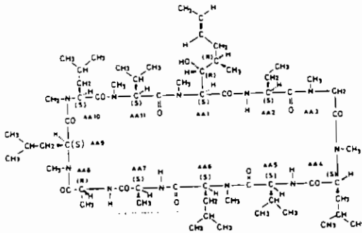
شكل (١٤٤) : تركيب السيكلوسبورين
