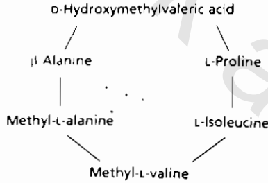
Destruxin B ( Metarhizium anisopliae )
