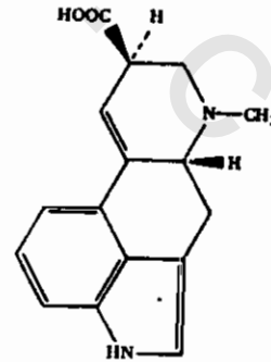
شكل (٣٠٤) : التركيب الكيميائى لحمض الليسرجيك.
