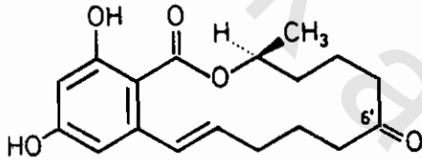
Zearalenone
