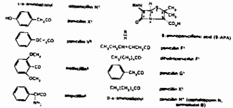
(شكل ٤٣٠) : بعض مركبات البنسلين.
