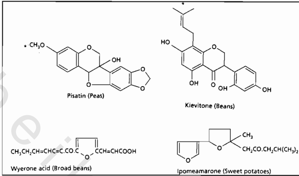
شكل (٤٤٤) تركيب بعض الفيتوالكسينات.
