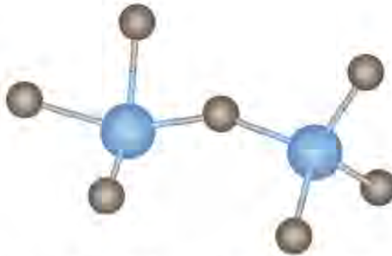
الشكل رقم (٧؁ ١). وءءاء بناء الزفولفء. اءئان من رباعفاء SiO_4/AlO_4 مءصلان بفءاسم الركن.
