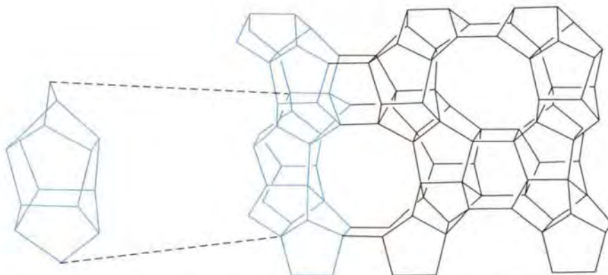
الشكل رقم (٧، ١١). وحدة بتاسيل مع شريحة من التركيب ZSM-5 موضحة سلسلة متصلة من وحدات بتاسيل.
