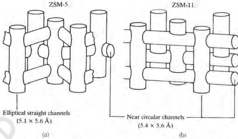
الشكل رقم (١٣، ٧). أنظمة اتصال قنوات دائرية داخلي في ZSM-11 و ZSM-5.
