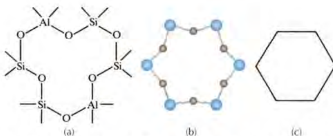
الشكل رقم (٧,٣). (a) حلقة 6 تحتوي على ذرتي Al وأربع ذرات Si (b) نموذج حاسوب للحلقة 6 و (c) نسخة مختزلة من نفس الحلقة 6.
