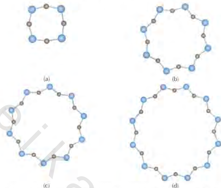
الشكل رقم (٩، ٧). نماذج حاسوب لأحجام نافذة متنوعة في الزبوليتات (a) الحلقة 4- (b) الحلقة 8- (c) الحلقة 10- و (d) الحلقة 12-.
