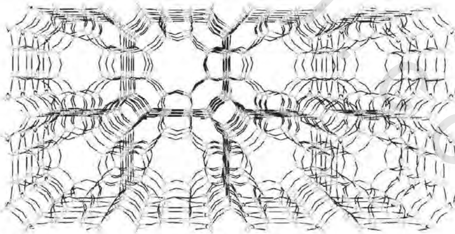
الشكل رقم (٧، ١٠). نموذج بالحاسوب لتركيب الزيوليت (LTA) A موضحاً القنوات ونوافذ الحلقة 8-.
