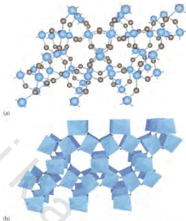
الشكل رقم (٧,٢). تركيب الكوارتز (a) كنمثيل كرة وقضيب (b) كرباعيات [\text{SiO}_4] متصلة.
