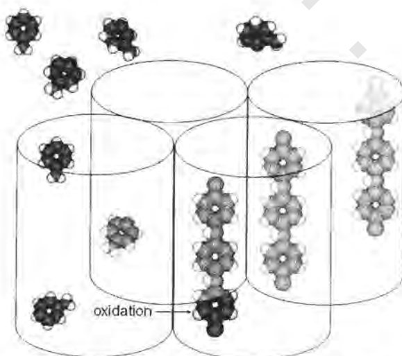
الشكل رقم (٧، ٢٣). كبسلة الأنيلين وتكوين بولي أنيلين في MCM-41.
