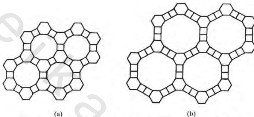
الشكل رقم (٧، ٢٤). رسومات إسقاط تركيبية تخطيطية لـ (a) ALPO-5 و (b) VPI-5.
