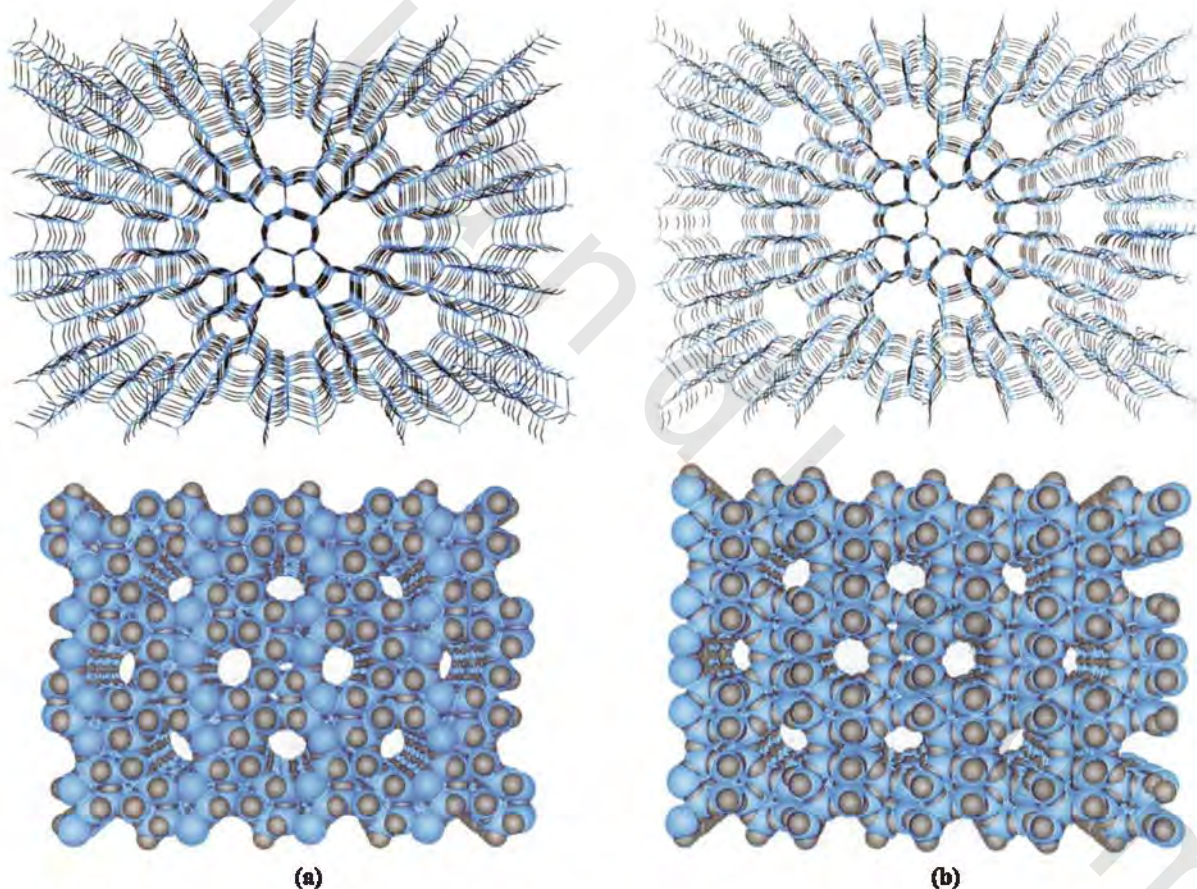
الشكل رقم (٧، ١٢). (a) نموذج بالحاسوب لـ ZSM-5 متعامد الأضلاع، موضحاً القنوات الأهلجية العمودية على طول الاتجاه y (b) نموذج بالحاسوب لـ ZSM-11 مظهراً القنوات العمودية القريبة إلى الدائرية التي تجرى على طول الاتجاهين x و y في بلورات رباعي الأضلاع. يمكن وصف كلا التركيبين كرسومات خطية ومع أنصاف أقطار فان درفالس لها.
