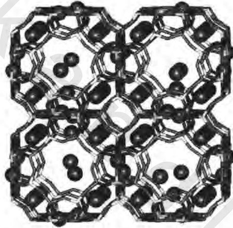
الشكل رقم (٧،٨). إطار ومواقع كاتيونية من الشكل Na^+ من الزيوليت (LTA). شاهد إدراج اللون في صفحة 356 (Courtesy of Dr. Robert Bell, Royal Institution of Great Britain, London).
