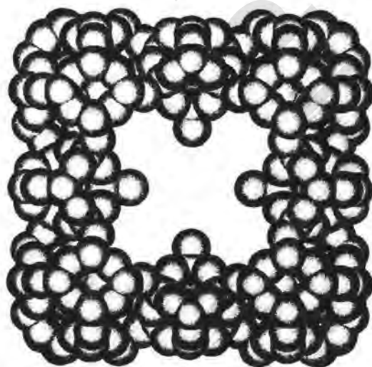
الشكل رقم (٧، ٢٥). إطار الجالوفوسفات المشيد، كلوفيريت، ممثلة على هيئة كرات مظلمة بأنصاف أقطار فان درفالس. (From C.R.A. Catlow 9ed.) (1992) Modelling of Structure and Reactivity in Zeolites , Academic Press, London. (Reproduction with permission of Academic Press Ltd.)
