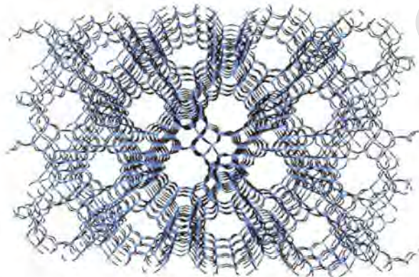
الشكل رقم (١٤، ٧). تركيب فاجاسيت مكبي موضحاً القنوات التي تقع موازية لكل من الأقطار الوجيهة (تدخل قنوات الأكسجين في هذا النموذج).
