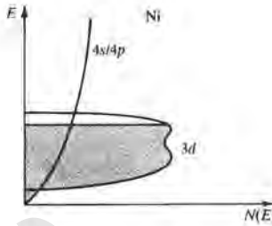
الشكل رقم (٤, ٣). تركيب النطاق للنكل. لاحظ شكل نطاق 3d.
