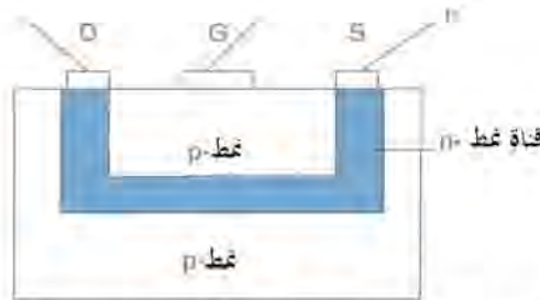
الشكل رقم (١٢، ٤). رسم تخطيطي لـ FET نصف أقطاب المصدر S، التصريف D والبوابة G.
