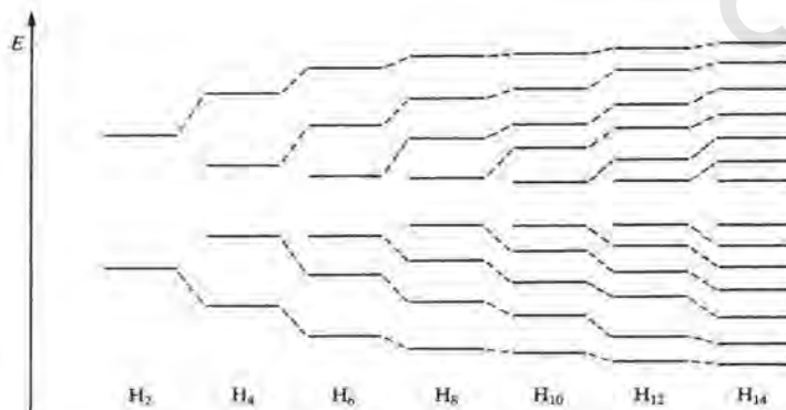
الشكل رقم (٤, ٦). طاقات مدارية لسلسلة N من ذرات الهيدروجين كلما تزايدت N .
