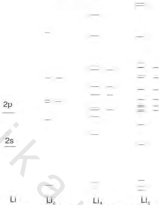
الشكل رقم (٤,٧). مستويات 2s و 2p لذرة Li وللسلاسل من ذرات Li 2، 4 و 6.
