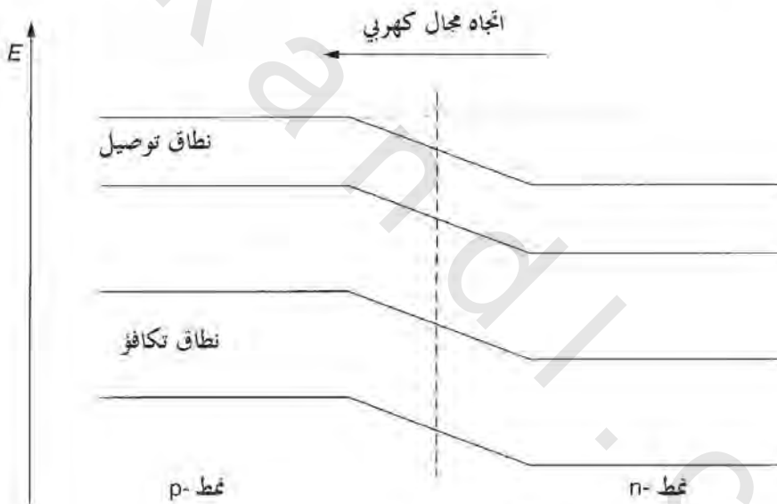
الشكل رقم (٤, ١١). تقوس، مستويات الطاقة عبر وصلة p-n.
