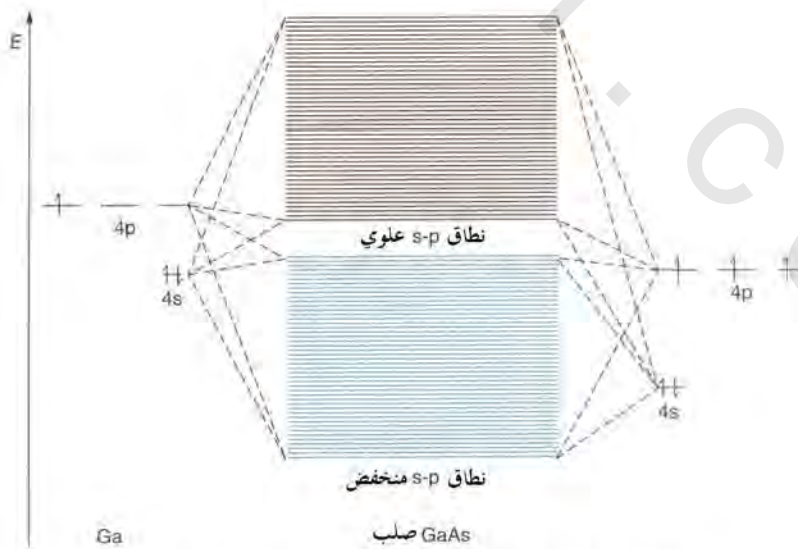
الشكل رقم (٤, ١٣). مخطط مستوى طاقة مدارية لأرزنيذ الجاليوم.
