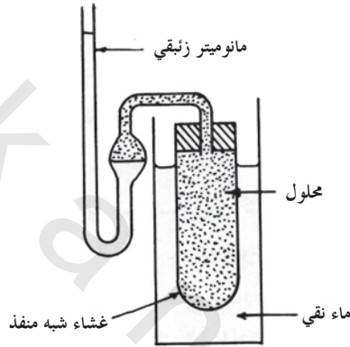
الشكل (٤-١٧). رسم تخطيطي لأسموميتر بسيط.
