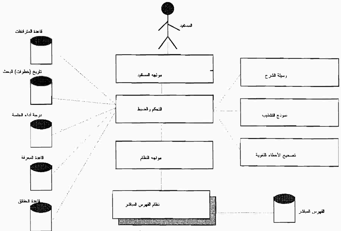
شكل (١) معمارية للنظام الخبير
