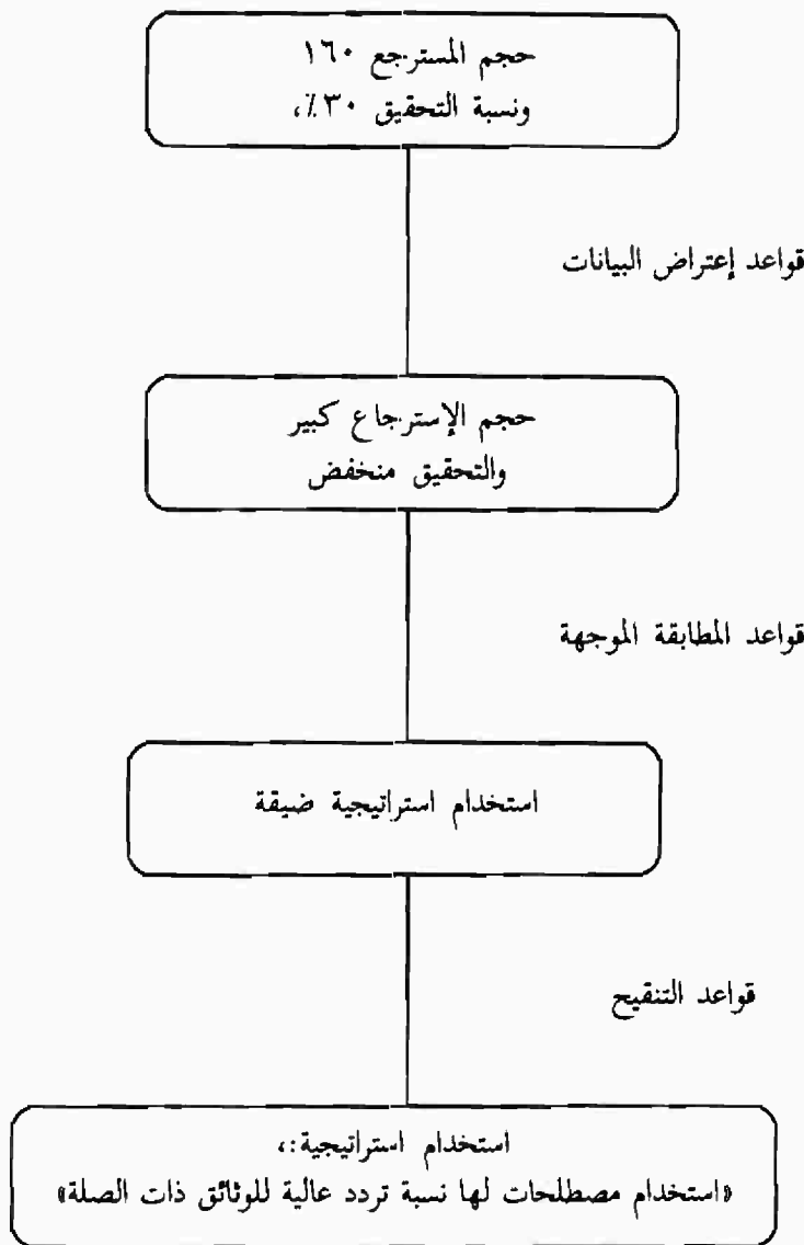
شكل ٢ . سلسلة قواعدا الاستدلال.
