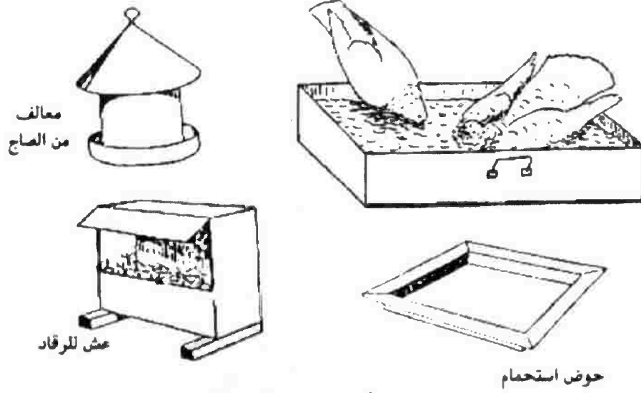
شكل ( ١٩ ) : المعدات والتجهيزات اللازمة لمسكن الحمام
