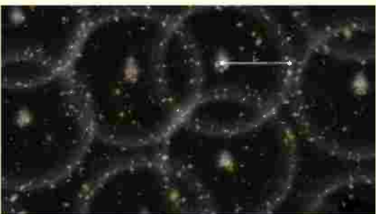
معرفة المسافات من خلال مقياس باربيون سوف تساعد في التأكد من الخصائص الأساسية للكون
