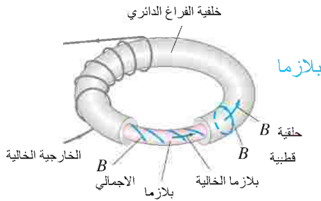
الشكل 31 - 12 مخطط للتوكاماك يرينا المجال المغناطيسي الكلي \vec{B} الناتج من تيار خارجي والتيار في البلازما نفسها.
