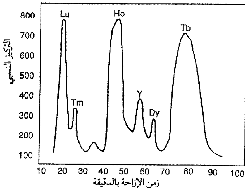
شكل ٤ - ٣ فصل العناصر اللانثانية.
