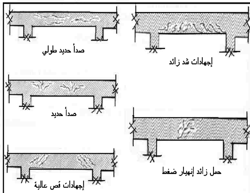
عيوب الكمرات
