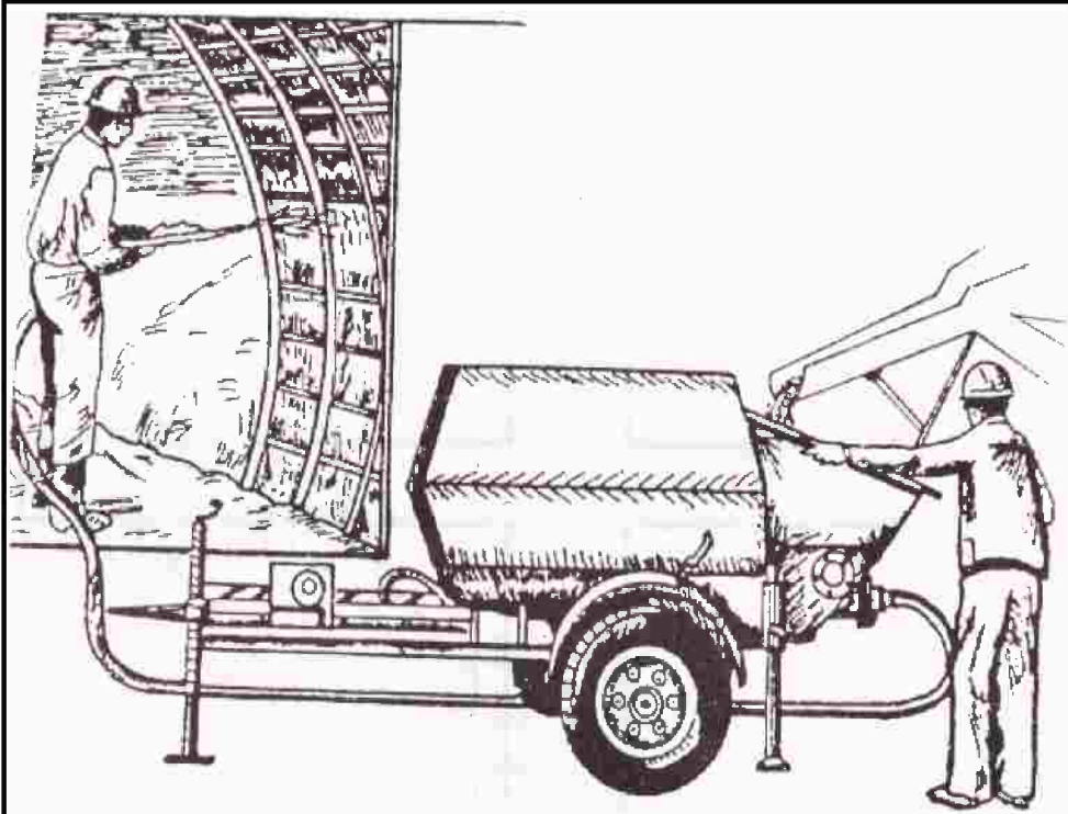
صورة توضح عمل الخرسانة بواسطة مدفع الخرسانة في أحد الانفاق والتي تصب الخرسانة فيها بدون عمل فرم خشبية لها كذلك تستخدم هذا النوع من الصب في أعمال لترميمات والقمصان SPRAYED CONCRETE BY CEMENT GUN & SHOUTCRE
