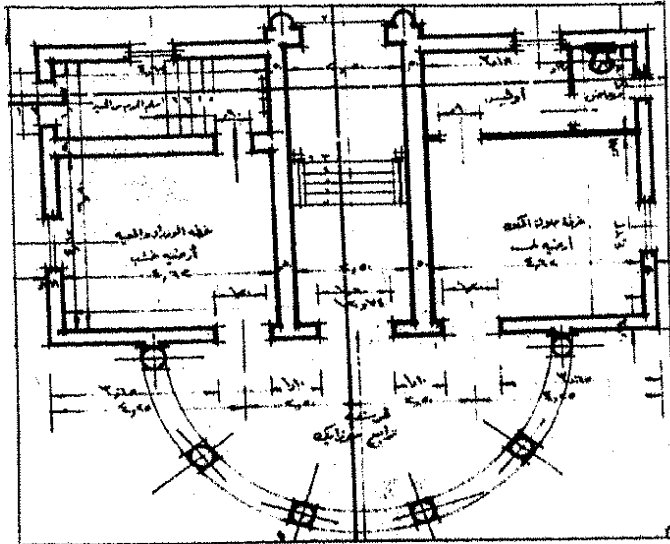
مسقط الدور الاول للكشك المكي ويرى في اليمين غرفة جلالة الملك وفي اليسار غرفة الوزراء والمعية
