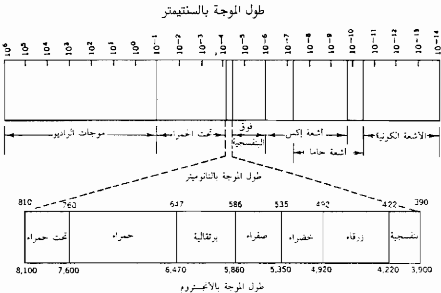
شكل ملحق (٦-١): أنواع الأشعة الكهرومغناطيسية وأطول موجاتها.
